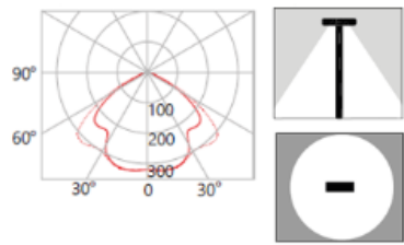
park light distribution | rozsył światła
