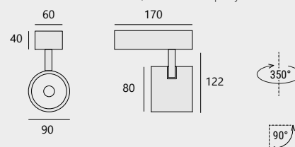
surface mounted/montaż nastropowy
