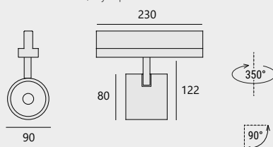
track 230V/szynoprzewód 230V
