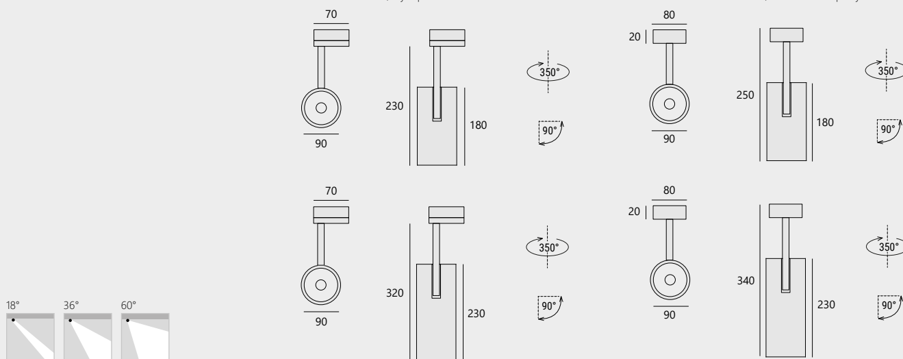
track 230V/szynoprzewód 230V
