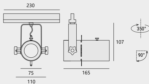
track 230V/szynoprzewód 230V
